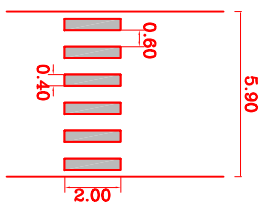
DETALHE 2 FAIXA DE PEDESTRE RUA SÃO SEBASTIÃO ESQUINA COM A RUA SÃO FRANCISCO
