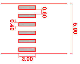
DETALHE 1 FAIXA DE PEDESTRE RUA SÃO SEBASTIÃO ESQUINA COM A RUA ADOLFO THOMAZ DE AQUINO
